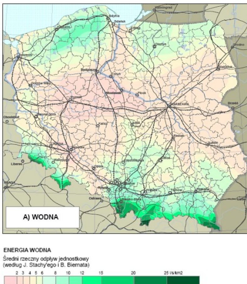
Rysunek 10 Energia wodna
