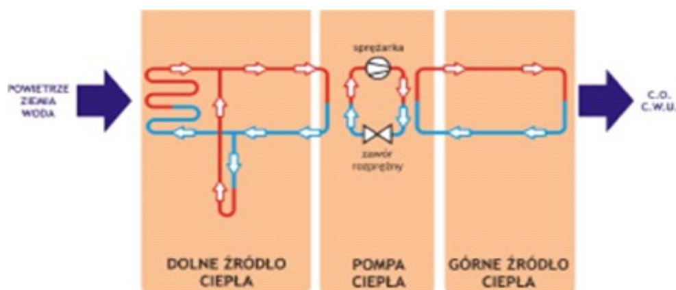
Rysunek 12 Zasada działania pompy ciepła Źródło: Instytut Energetyki Odnawialnej (EC BREC IEO)
